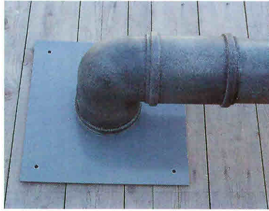
Fastgørelse af ålepas udført i plastør kan ske ved at montere en rørflange på styrtvæggen.
