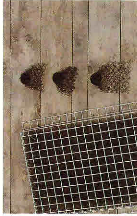
Stoppematerialet skal føres igennem hullerne og have forbindelse med selve passet, her er Enkamaten fastsyet i en trådkurv.
